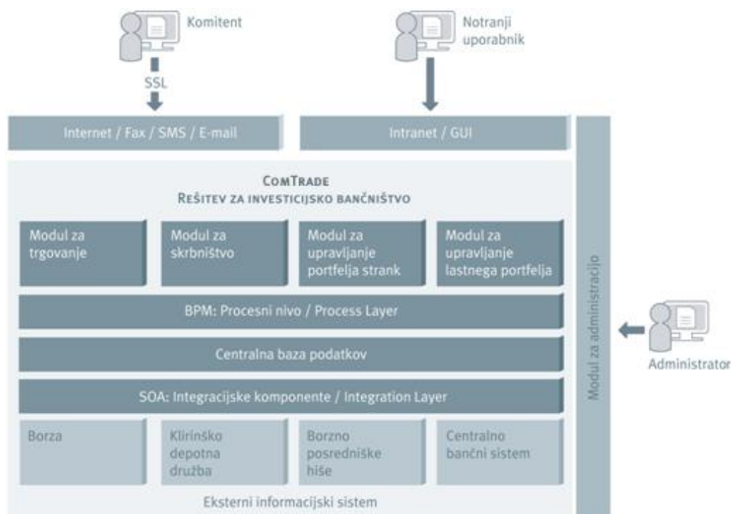
Slika 1: Arhitektura rešitve za investicijsko bančništvo
