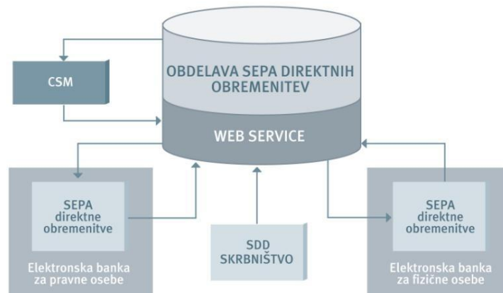
Slika 2: Shema ComTradeove rešitve za SEPA DD
